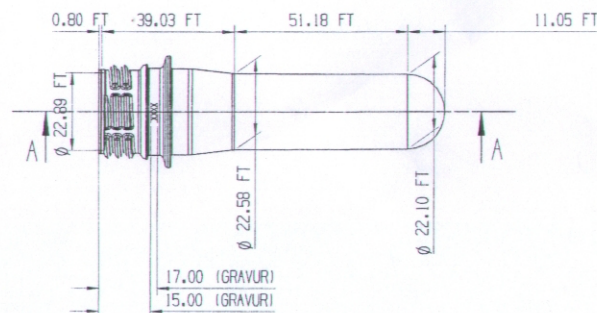
ANSICHT FORMTRENUNG M 1:1
